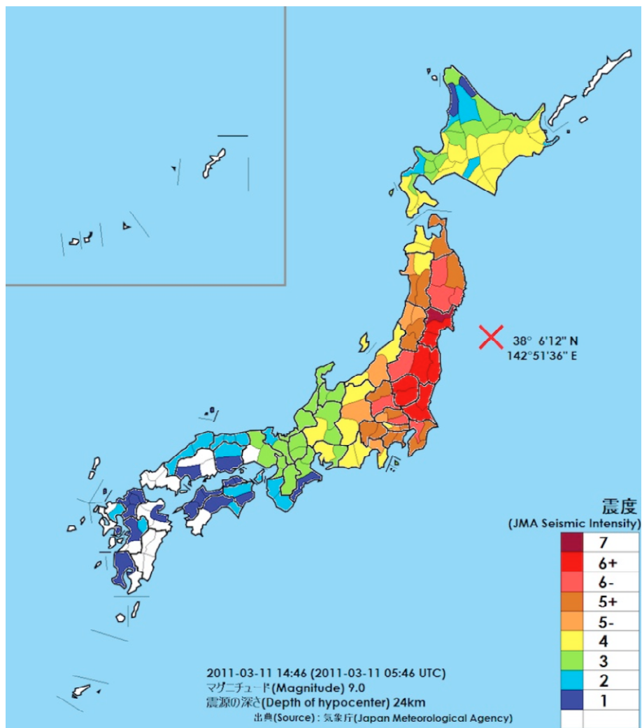
図：東日本大震災・各地の震度（出典：復興対策本部資料より）
